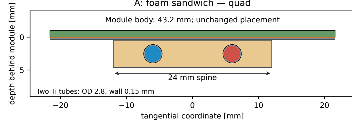
A: foam sandwich — quad
