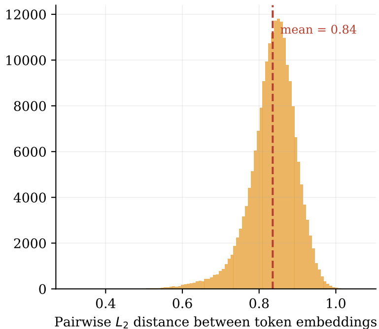
Llama-3 8B
