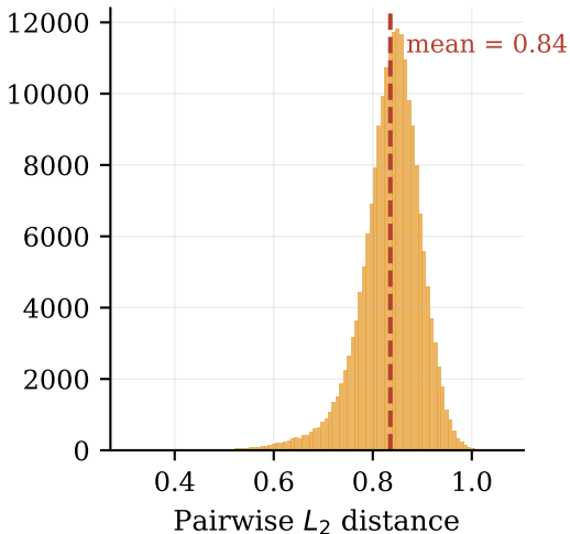
Llama-3 8B
