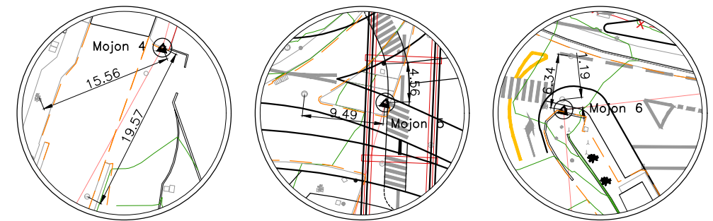
REFERENCIA DE MOJONES ESC: 1:500
