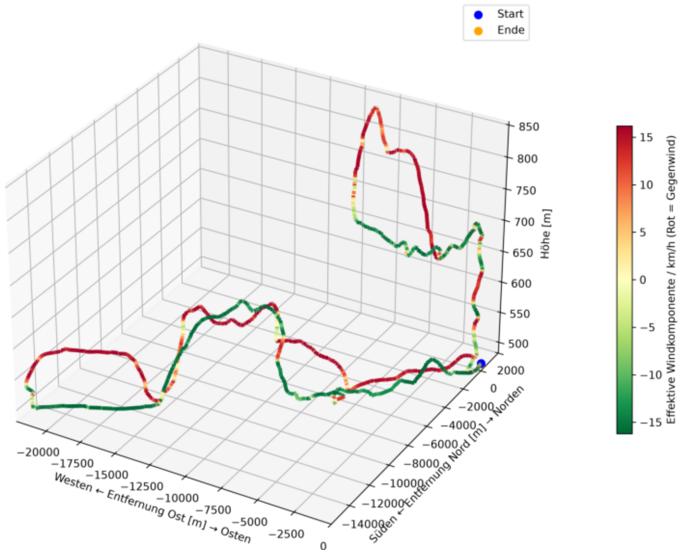
3D-Streckenprofil mit farbkodiertem Windeinfluss
