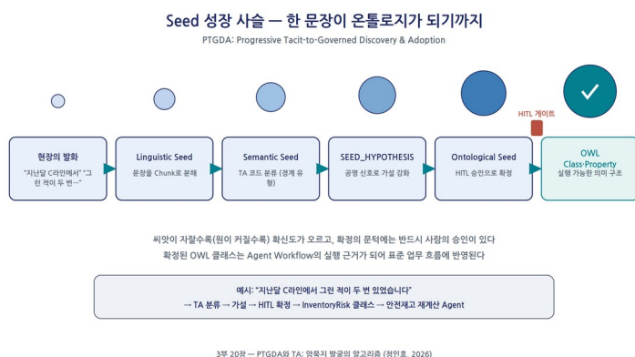
그림 19-5. Seed 성장 사슬 — 언어가 스키마가 되기까지
