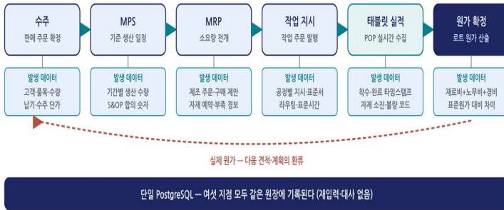
그림 13-2. 제조 데이터 흐름 — 수주에서 원가까지
