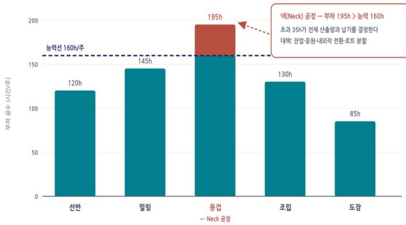
그림 4-3. 공수 산적표 — 능력선과 부하, 넥 공정
