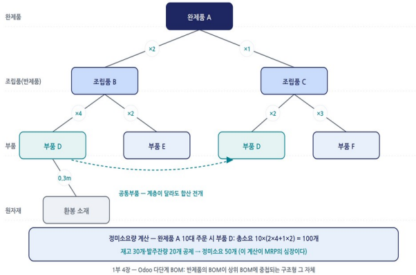
그림 4-1. 구조형 부품표(BOM) 트리와 정미소요량 계산
