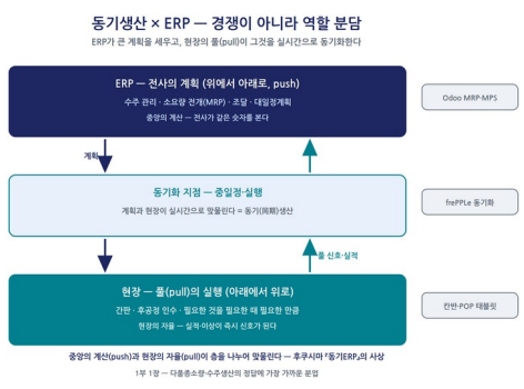
그림 1-2. 동기생산(간판) × ERP의 역할 분담
