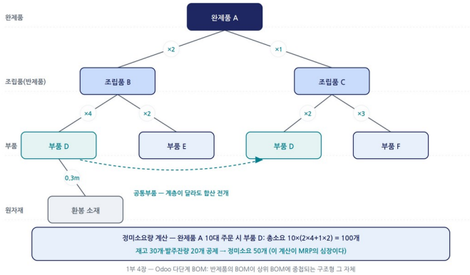
그림 4-1. 구조형 부품표(BOM) 트리와 정미소요량 계산
