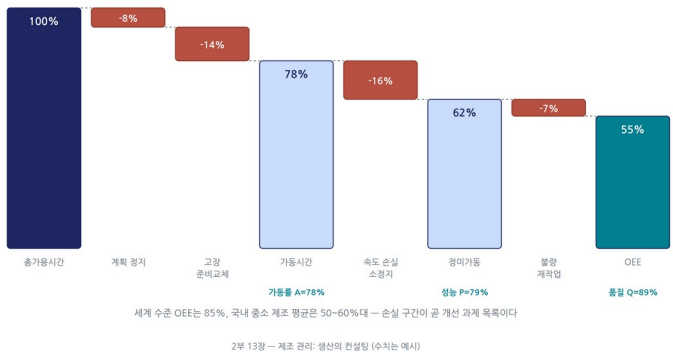
그림 13-1. OEE 폭포 — 100%는 어디서 깎여 나가는가 (수치는 예시)
