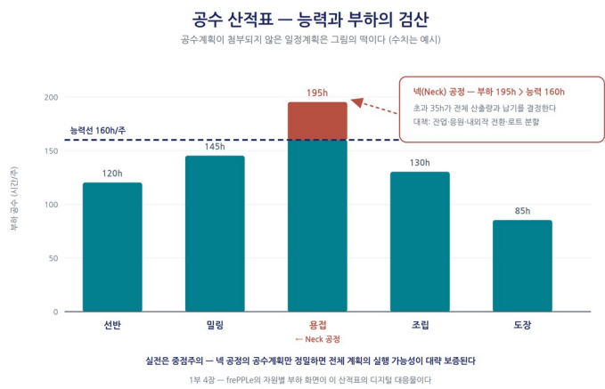
그림 4-3. 공수 산적표 — 능력선과 부하, 넥 공정
