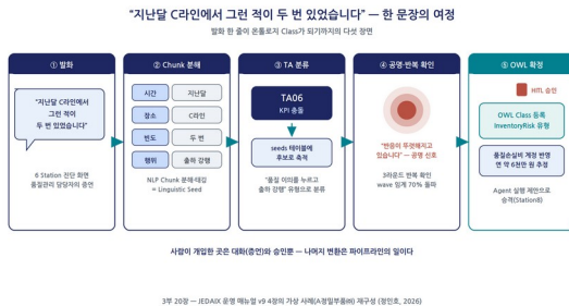
그림 19-6. 한 문장의 여정 — 발화에서 OWL 확정까지
