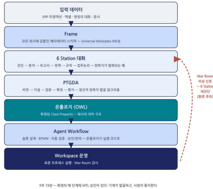
그림 19-1. 온톨로지-지식그래프전체 파이프라인 — 말에서 실행까지
