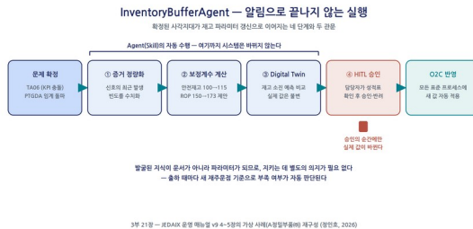
그림 20-2. InventoryBufferAgent 실행 순서 — 증거 정량화, 보정 계산, 시물레이션, 사람의 승인
