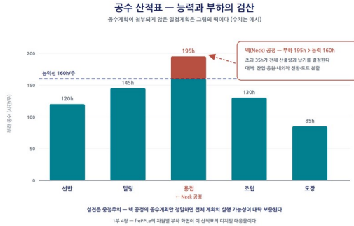
그림 4-3. 공수 산적표 — 능력선과 부하, 넥 공정
