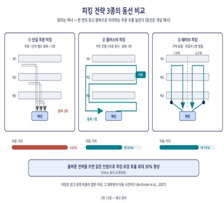
그림 12-3. 피킹 전략 3종의 동선 비교 — 단일·클러스터·웨이브 (동선은 개념 예시)
