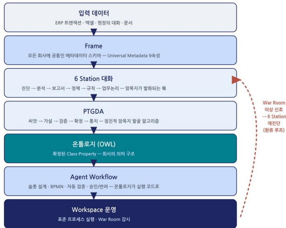
JEDAIX 전체 파이프라인 — 대화가 온톨로지가 되고, 온톨로지가 실행이 된다
