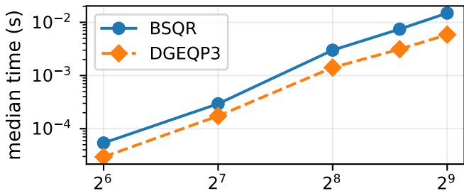
orthonormal_rows | BLAS=1
