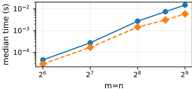
orthonormal_rows | BLAS=1
