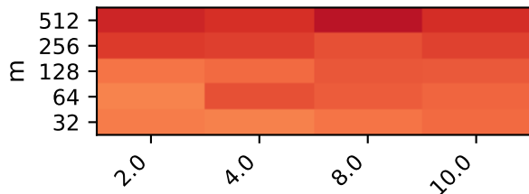
orthonormal_rows | BLAS=1
