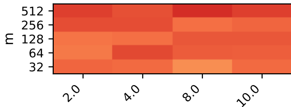
orthonormal_rows | BLAS=4
