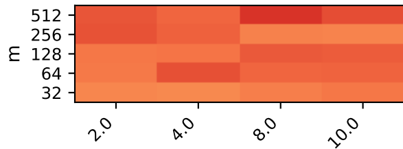
orthonormal_rows | BLAS=1
