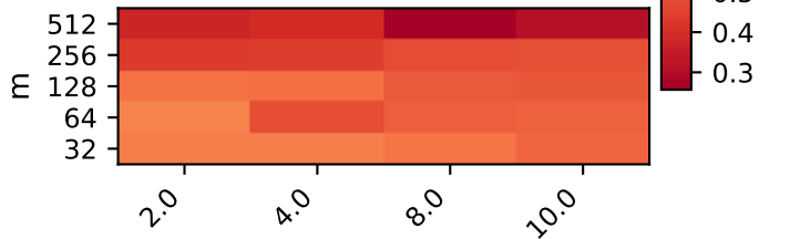
orthonormal_rows | BLAS=4
