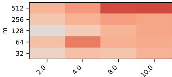
Orthonormal rows | BLAS=1
