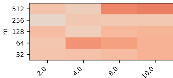
Orthonormal rows | BLAS=4
