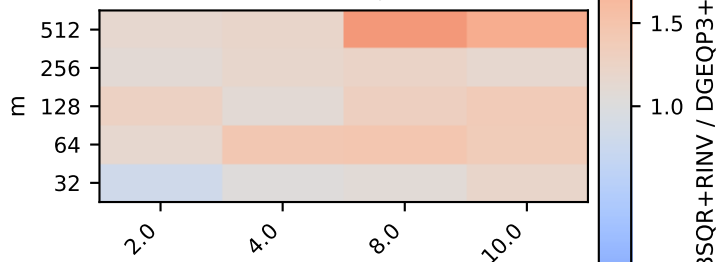
Orthonormal rows | BLAS=4
