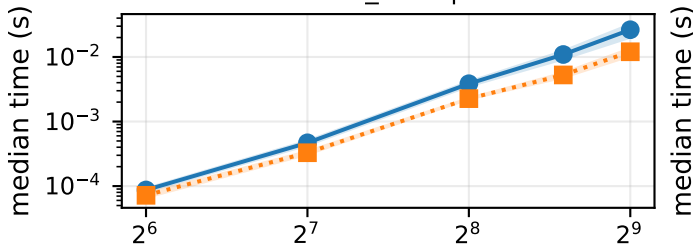
orthonormal_rows | BLAS=1
