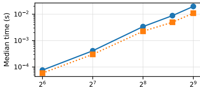
Orthonormal rows | BLAS=4
