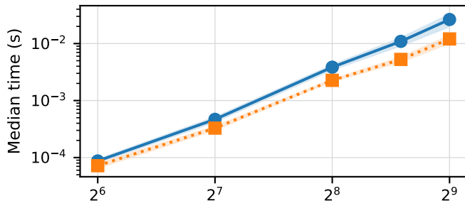
Orthonormal rows | BLAS=1
