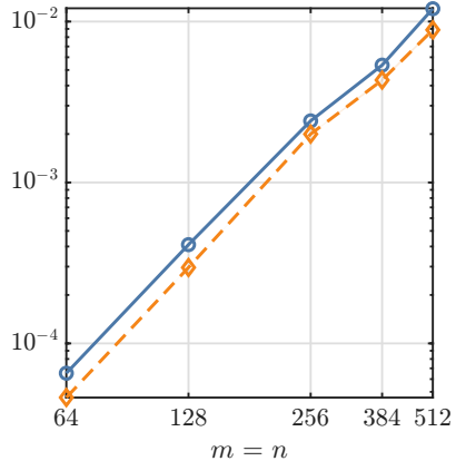
Orthonormal rows
