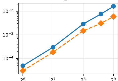
orthonormal_rows, BLAS=8
