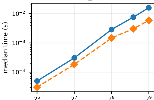
orthonormal_rows, BLAS=1
