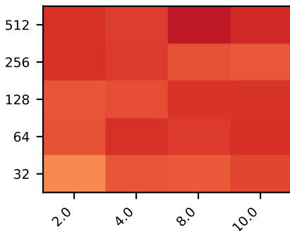
orthonormal_rows, BLAS=8
