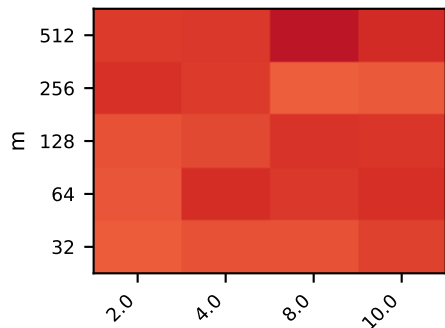
orthonormal_rows, BLAS=1
