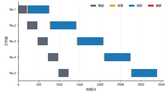
图 8 采掘接续时序甘特图
