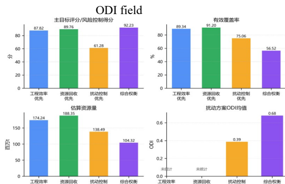
图 7 多目标规划模式指标对比结果
