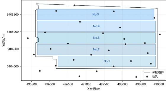
图 5 采区规划布局结果
