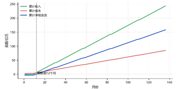
图 10 采掘接续方案现金流分析结果
