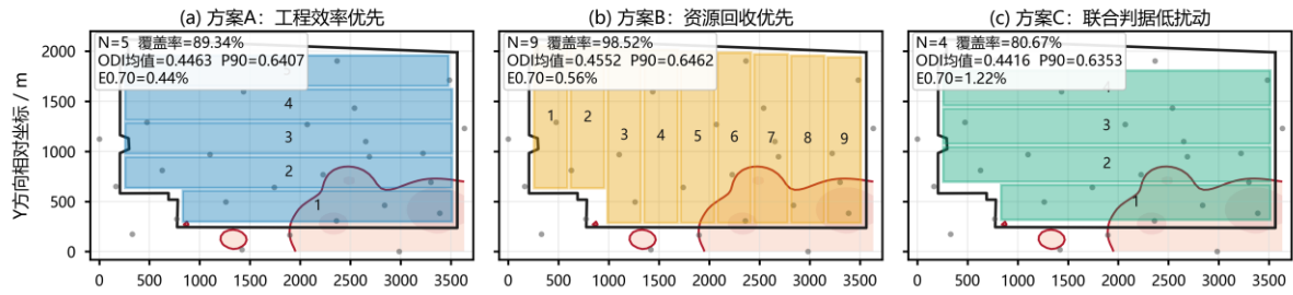
图 5 A/B/C 候选方案工作面布局与 ODI 高值区叠置对比图 Fig.5 Comparison of A/B/C candidate layouts overlaid with high-ODI zones
