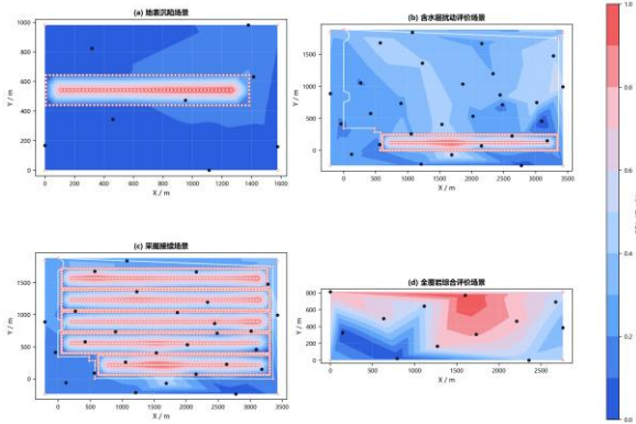
图 4 多场景 ODI 分布结果对比图
