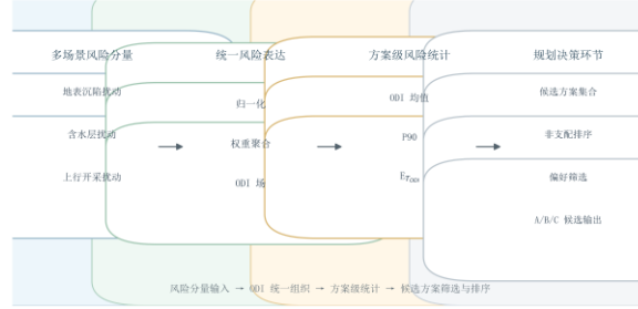
图 1 ODI 风险约束逻辑示意图
