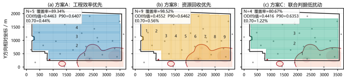
图 5 A/B/C 候选方案工作面布局与 ODI 高值区叠置对比图
