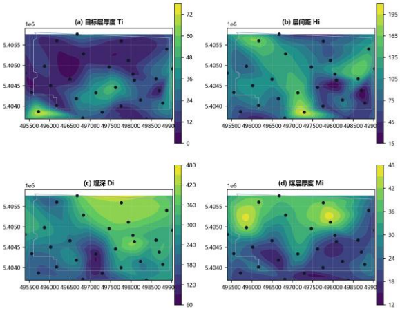
图 3 研究区主要地质参数场分布图
