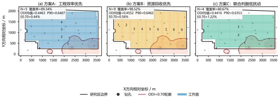
图 5 A/B/C 候选方案工作面布局与 ODI 高值区叠置对比图
