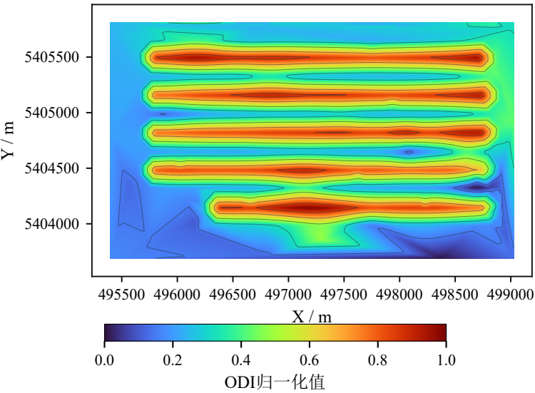
(c) 上行开采扰动
