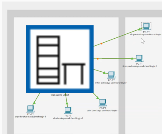
Рис. 3: Размещение в физической рабочей области серверной с подключением оконечных устройств на территории Донская
