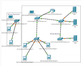
Рис. 8: Логическая топология
