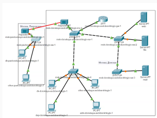
Рис. 11: Схема сети с учётом физических параметров сети в логической рабочей области
