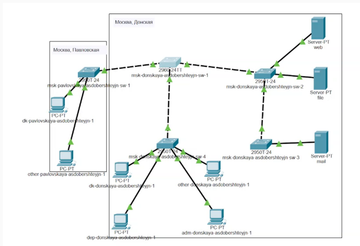
Рис. 1: Схема сети L1
