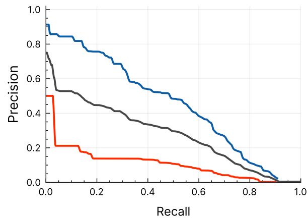
YOLO26
