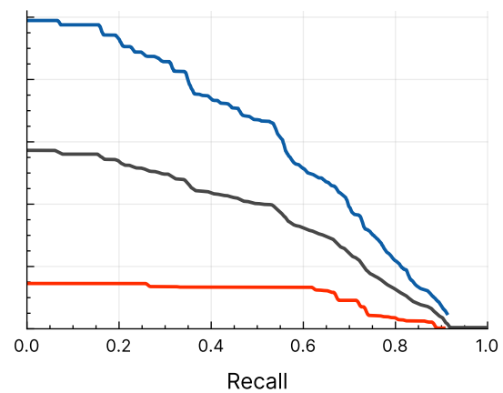
YOLO26 + DraxNet
