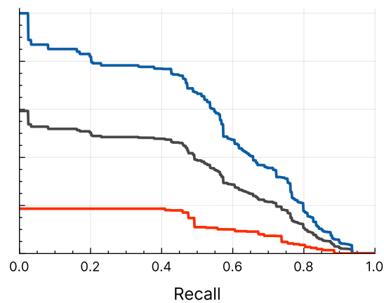
YOLO11n
