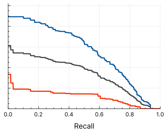
YOLOv8n
