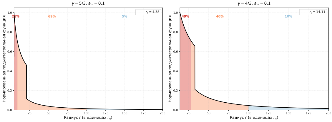
Рис. 2: Подынтегральная функция 4\pi r^2 \rho v_{\text{acc}}^2(r) из (19), нормированная на своё максимальное значение, как функция r (в единицах r_g ) при a_\infty = 0.1 . Левая панель: \gamma = 5/3 ; правая панель: \gamma = 4/3 . Закрашенные области выделяют вклады трёх радиальных интервалов: [r_c, 2r_a] (область акустического горизонта), [2r_a, r_B/2] (промежуточная зона) и [r_B/2, r_B] (внешняя зона). Вертикальная штриховая линия отмечает r_c . Численные доли вклада каждого интервала в полный момент инерции I указаны на вставках.
