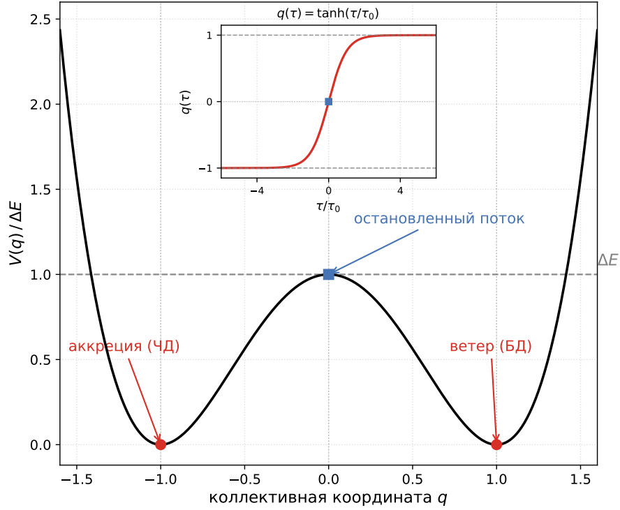
Рис. 3: Модельный потенциал двойной ямы V(q) = \Delta E(1 - q^2)^2 из (20) (сплошная чёрная кривая); потенциал V дан в единицах \Delta E , коллективная координата q безразмерна. Минимумы при q = \pm 1 соответствуют аккреционной и ветровой ветвям; максимум V(0) = \Delta E при q = 0 — остановленному потоку. Пунктирная горизонтальная линия отмечает уровень \Delta E . Вставка: инстантонная траектория q(\tau) = \tanh(\tau/\tau_0) как функция евклидова времени \tau в единицах \tau_0 .
