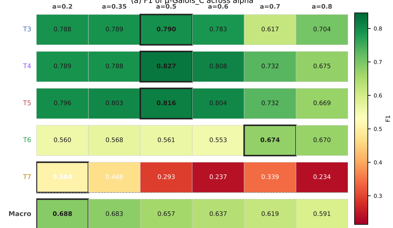
(a) F1 of \mu -Galois_C across alpha
