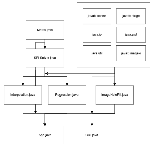
Gambar 3.2: Jalur Dependensi
