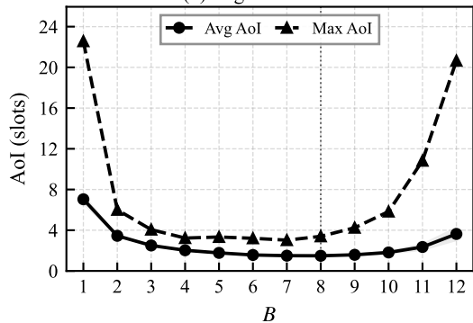
(d) Avg and Max AoI
