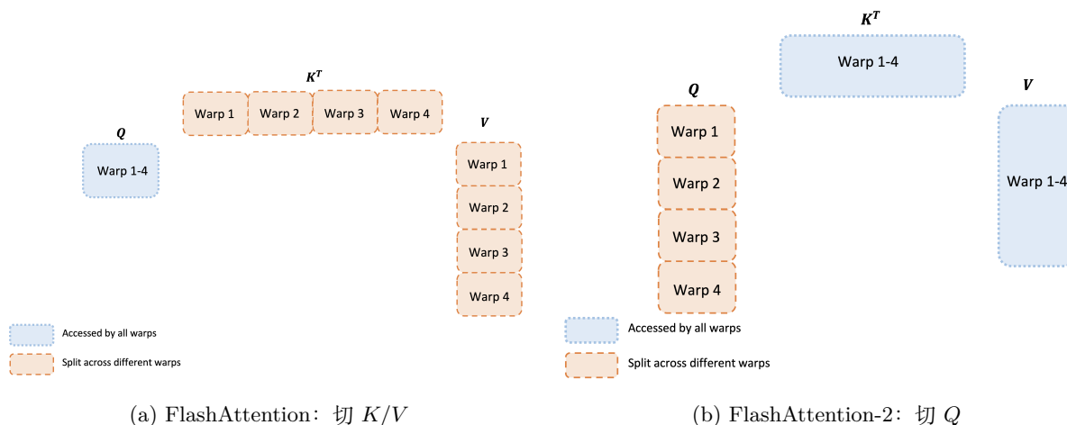
论文 Fig. 3: Dao. FlashAttention-2: Faster Attention with Better Parallelism and Work Partitioning . ICLR 2024. 蓝: 所有 warp 共享; 橙: 切到不同 warp。
