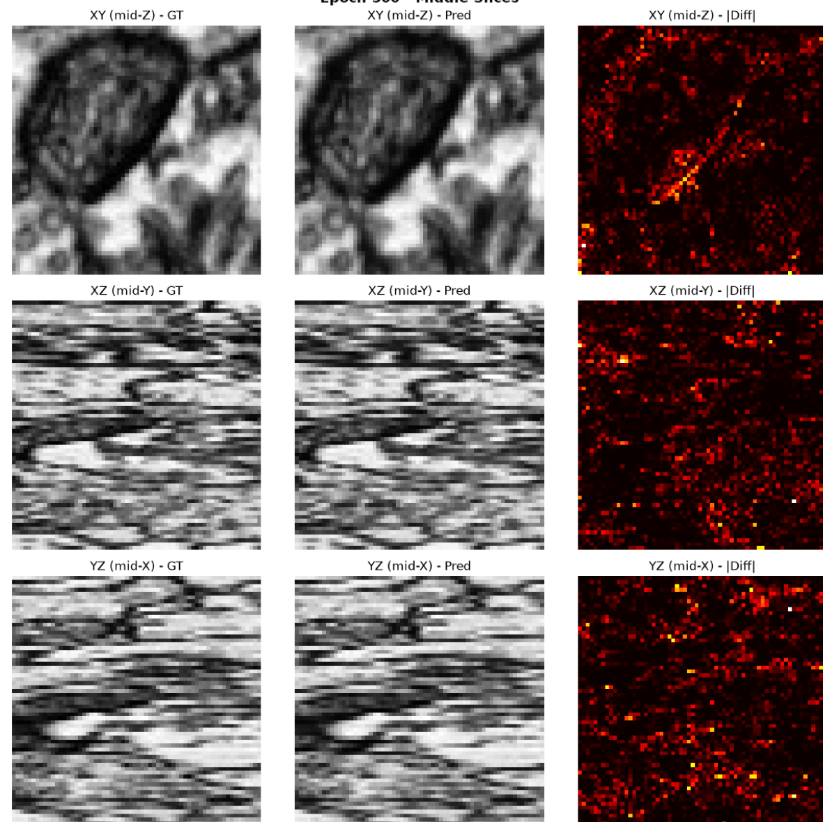
(d) b_231 — vol_PSNR = 40.23 dB
