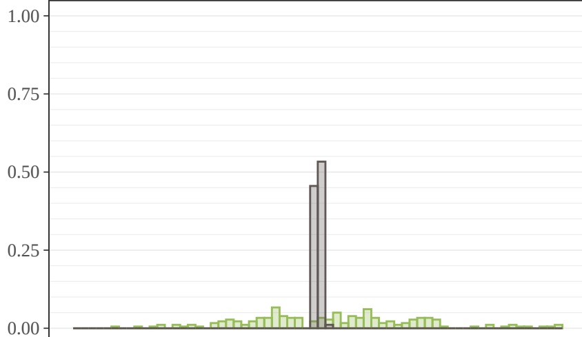
GPT-3.5-Turbo
