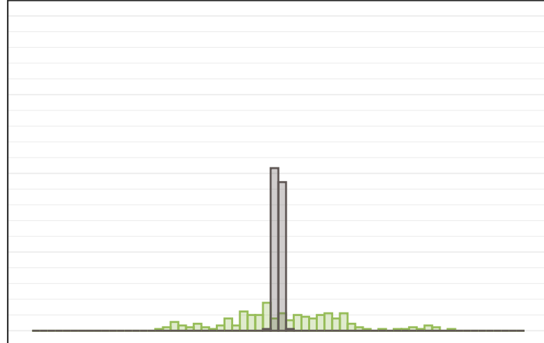
GPT-4o
