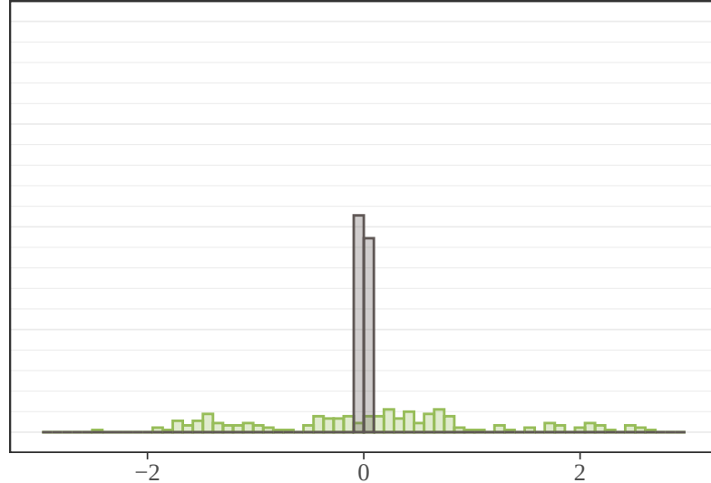
GPT-5-Nano
