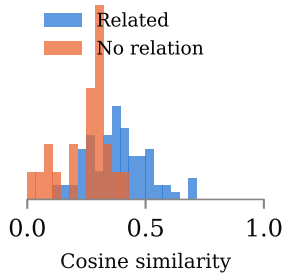
SBERT
