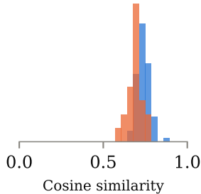
Gemini emb.
