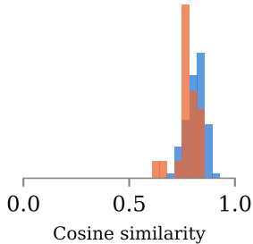
BERT
