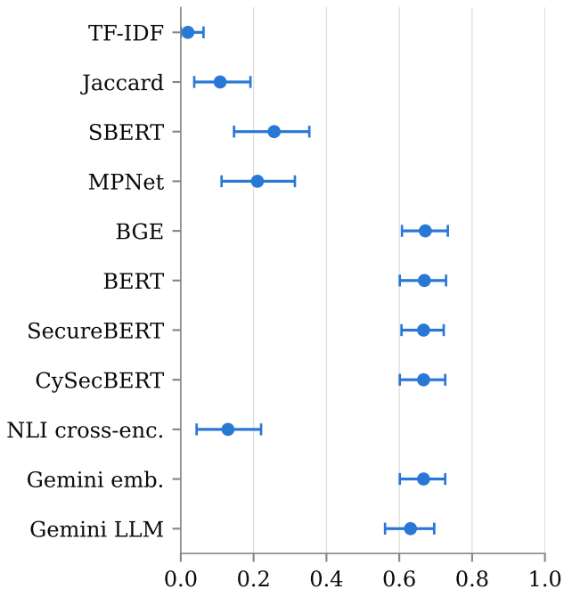
Pair-detection F1
