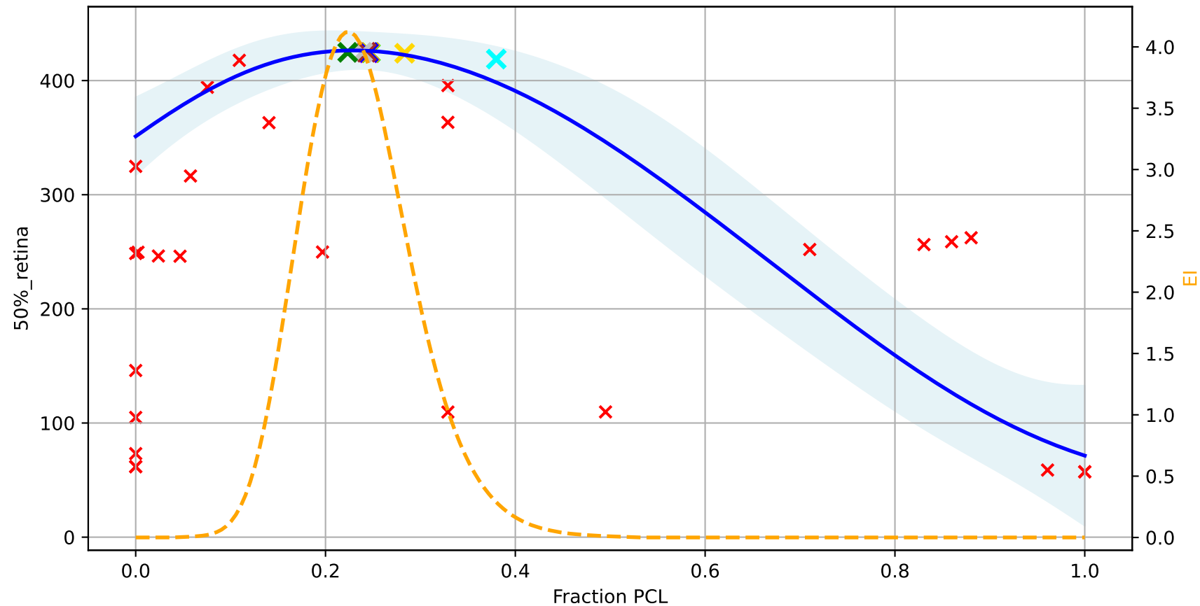
GP Posterior + EI Slice at Total Radius = 0.0015
