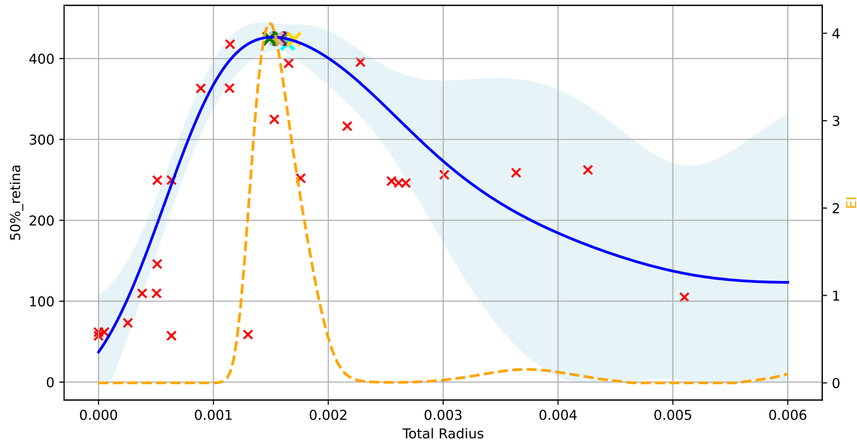
GP Posterior + EI Slice at Fraction PCL = 0.22
