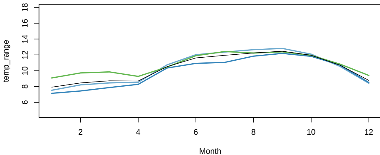
temp_range Group 11
