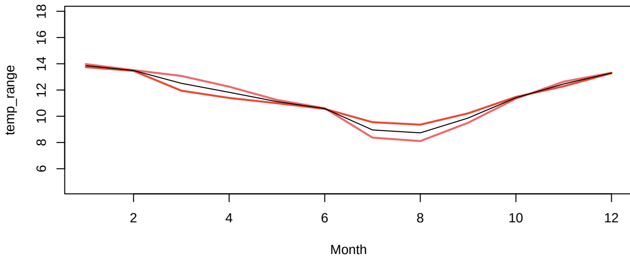
temp_range Group 3
