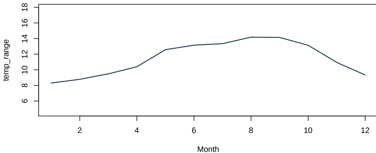
temp_range Group 10
