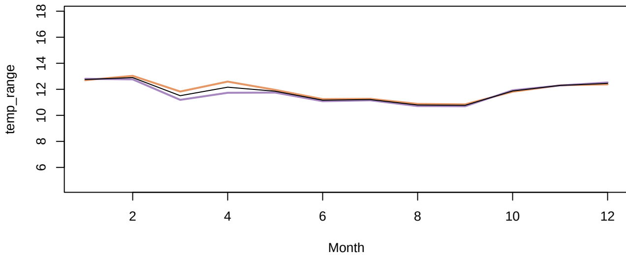
temp_range Group 2
