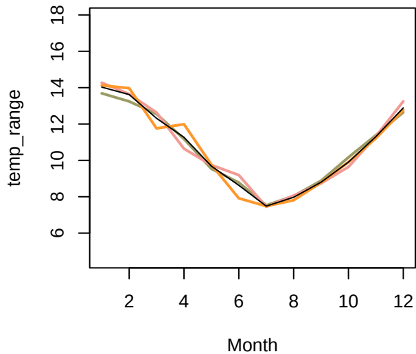
temp_range Group 5
