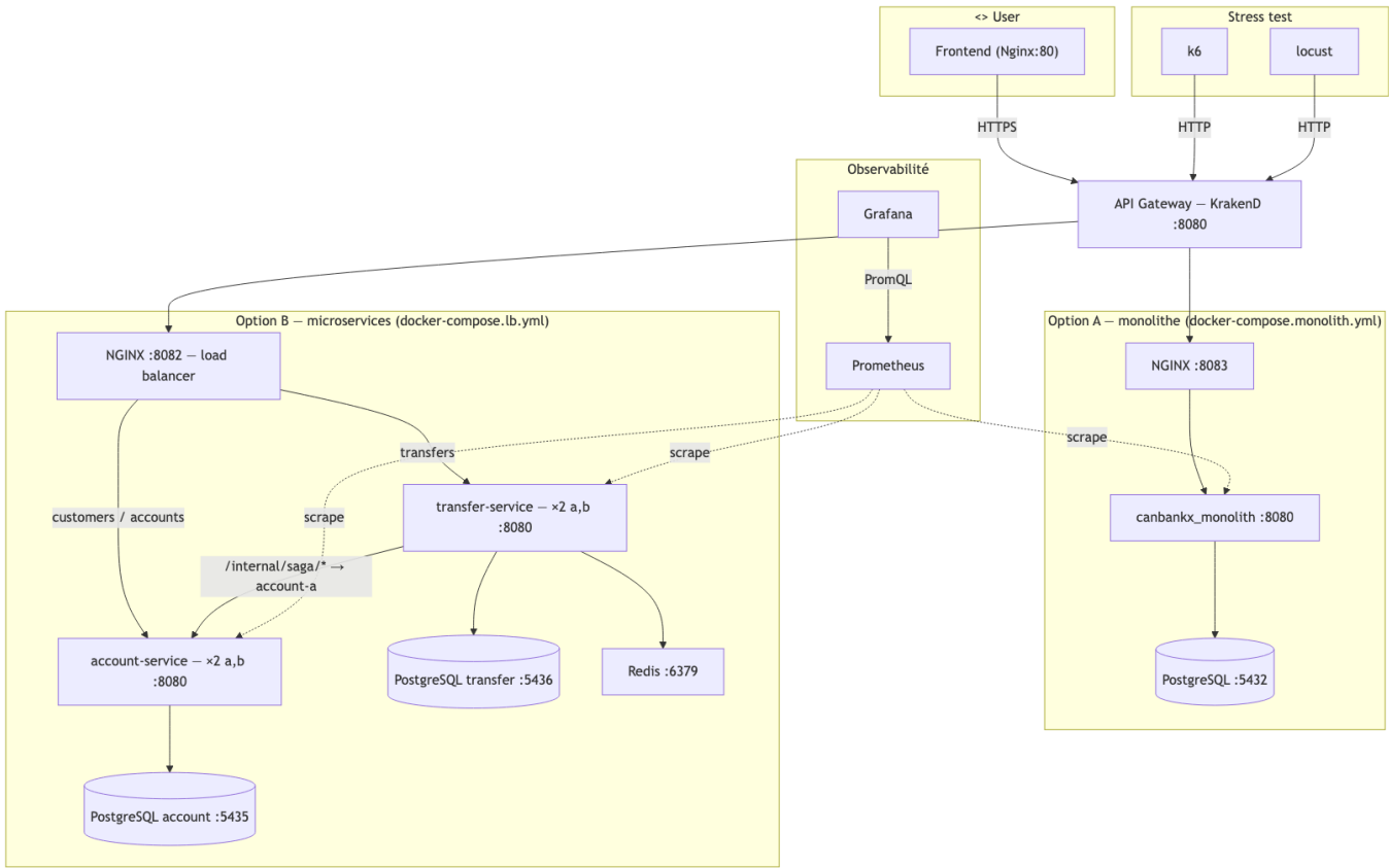
Figure 12. Diagramme Déploiement — Monolith et Microservices (style Test1)
