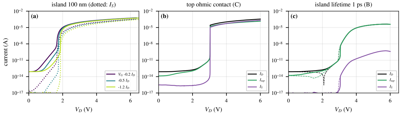
Fig. 9. 가로 PNP 결합을 끊는 세 방법 ( R_{tap} = 10 k \Omega ). (a) 섬 폭 100 nm, V_G = -0.2/-0.5/-1.2 V (실선 I_D , 점선 I_S ): 왼쪽이 함께 켜진다. (b) 섬 윗면 ohmic contact(C): I_{tap} , I_S 가 동시에 점프. (c) 섬 lifetime 1 ps(B): 오른쪽만 래치하고 I_S 는 10^{-9} A 아래 (점선 down). 데이터: 1001/tap/TAPT_ISL_W100_L3_R7_R1e4_{UP_VGm0p2,UPDN_VGm0p5,UPDN_VGm1p2}.log, 1001/tap/TAPT_ISL_W30TC_L3_R7_R1e4_UD6S_VGm0p2.log, 1001/tap/TAPT_ISL_W30LK_L3_R7_R1e4_UD6S_VGm0p2_extract.dat.
