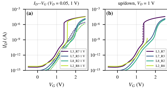
Fig. 6. 대농도차 split의 Id-Vg. (a) V_D = 0.05 V(점선)와 1 V(실선). (b) V_D = 1 V gate 왕복: L3 R7만 1.39/1.34 V의 gate 방향 래치와 hysteresis를 보인다. 데이터: 0928/idvg/IDVG_BIG_*_X50_{vd0p05,vd1}.log, 0928/idvg_return/IDVGR_BIG_*_X50_vd1.log.
