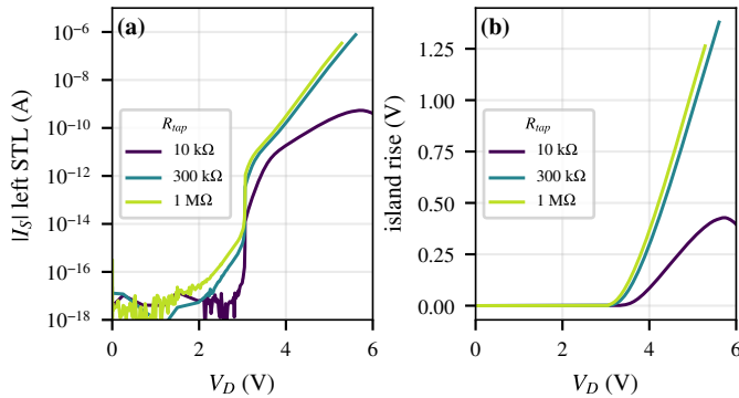
Fig. 10. B 구조(섬 lifetime 1 ps)에서 R_{tap} sweep (up). (a) 왼쪽 STL 전류 |I_S| , (b) 섬 전위 상승. 1 M \Omega 곡선은 5.28 V의 수치 오류 직전까지 표시. 데이터: 1001/tap/TAPT_ISL_W30LK_L3_R7_{R1e4_UD6S,R3e5_UD7S}_VGm0p2_extract.dat, 1001/tap/TAPT_ISL_W30LK_L3_R7_R1e6_UD7S_VGm0p2.log.
