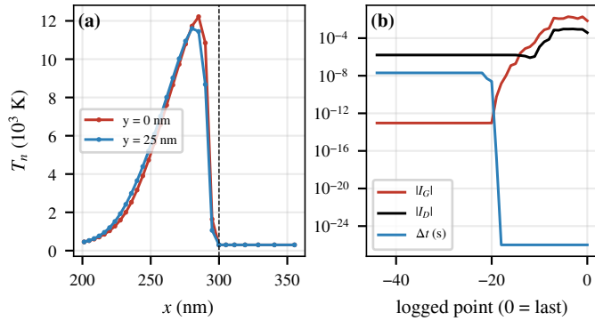
Fig. 23. hcte 실패 진단. (a) 5.25 V 전자 온도 T_n 단면 (표면, 중간 깊이; 점선: drain 경계). (b) R_{tap} = 1 M \Omega run의 마지막 45점; time step이 10^{-25} s로 붕괴한 뒤 |I_G| 가 10^{-13} 에서 10^{-3} A로 뛰는 가짜 점프. 데이터: 1001/tap/TAPT_ISL_W30LK_L3_R7_R1e6_RS50_NEWT_VGm0p2_UP_5p25.str, 1001/tap/TAPT_ISL_W30LK_L3_R7_R1e6_UD7S_VGm0p2.log.
