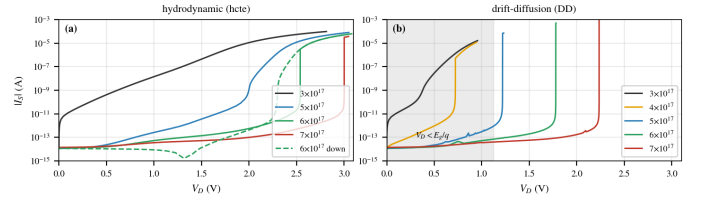
Fig. 11. Standalone 왼쪽 STL의 source 전류. (a) hcte: 3 \times 10^{17} , 5 \times 10^{17} 은 연속적으로 켜지고, 6 \times 10^{17} ( V_{LU} = 2.54 V, 점선: down sweep)과 7 \times 10^{17} (3.00 V)은 급격히 래치한다. (b) DD: 래치 전압이 0.7–0.8 V 낮고, V_D < E_g/q 영역의 래치(회색)는 DD의 impact ionization 과대평가로 본다. 데이터: 1001/tap/LEFTONLY_L135_P_{3,5,6,7}e17_UD6S_VGm0p2.log, 1001/tap/LEFTONLY_L135_P6e17_UD3_VGm0p2.log, 1001/tap/LEFTONLY_L135_P*_DD_UP4_VGm0p2.log.
