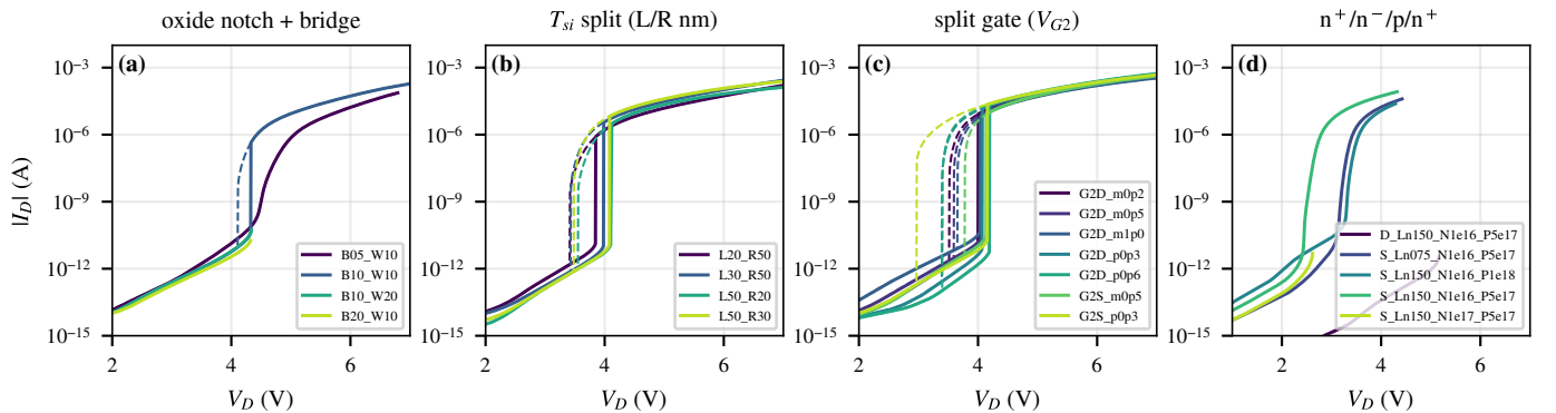
Fig. 5. 단일 body에서의 다른 분리 시도 (모두 래치 한 번). (a) 산화막 notch + Si bridge (B: bridge 두께, W: notch 폭, nm). (b) T_{si} split (왼쪽/오른쪽 두께 nm). (c) Split gate: 두 번째 gate 전압 V_{G2} (D: drain 쪽, S: source 쪽 gate). (d) n^+/n^-/p/n^+ (S/D: n^- 위치, Ln: n^- 길이 nm, N: n^- 도핑, P: p 도핑). 데이터: 0921/B*_W*_L5p0_R5p2.log, 0928/TSI_*.log, 0929/splitgate/SG_*.log, 1001/nnpn/NNPN_*.log.
