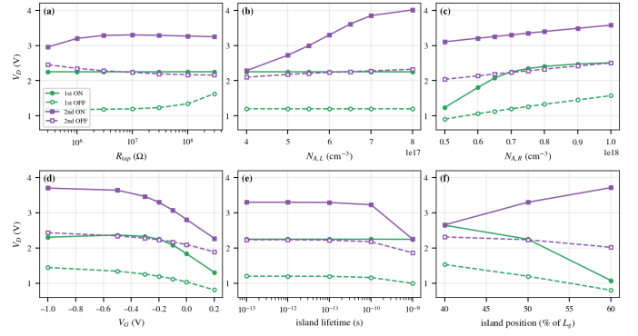
Fig. 17. 설계 손잡이: 두 래치의 ON(실선)/OFF(점선) 전압. (a) R_{tap} , (b) 왼쪽 body 도핑, (c) 오른쪽 body 도핑, (d) V_G , (e) 섬 lifetime, (f) 섬 위치. 데이터: 1007_ddsplit/ddsplitt_summary.dat (원본: 1007_ddsplit/DDS_*.log_tr.log, 텍 생성: 1007_ddsplit/make_ddsplit.py).
