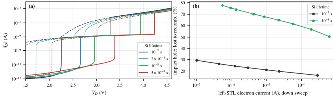
Fig. 16. Si lifetime와 급격한 꺼짐. (a) \tau_{Si} 에 따른 |I_D| - V_D : 수명이 짧을수록 두 번째 래치가 점프로 꺼진다 (OFF 폭 0.26→0.04 V). (b) Down sweep에서 왼쪽 STL의 impact 성공 중 재결합으로 잃는 비율. 데이터: 1007_ddsplit/DDS_{BASE,TE2em8,TE1em8,TE5em9}.log_tr.log, 1007_ddsplit/mech2_DD_S_{BASE,TE8}_SNAP.dat.
