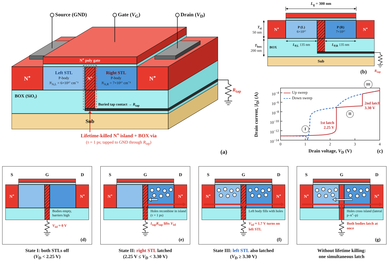
Fig. 1. 제안 소자와 동작 원리. (a) 왼쪽 STL(p-body 6 \times 10^{17} )과 오른쪽 STL(p-body 7 \times 10^{17} ) 사이의 lifetime-killed n^+ island를 BOX 관통 via와 R_{tap} 으로 접지한다. (b) 단면과 치수. (c) I_d - V_d 의 두 래치(I→II 2.25 V, II→III 3.30 V). (d)–(f) 각 상태의 body 정공. (g) 섬 lifetime을 줄이지 않으면 정공이 섬을 건너 두 body가 동시에 래치한다. 그림: docs/fig/paper/fig1_concept.png; (c)의 데이터: 1007_ddsplit/DDS_BASE.log_tr.log.
