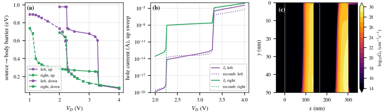
Fig. 14. .str 스냅샷 기반 메커니즘 (기준 소자, \tau_{Si} = 10^{-7} \text{ s} ). (a) STL별 source \rightarrow body 전자 장벽 (up 실선, down 점선): 각 래치에서 해당 STL의 장벽만 무너진다. (b) Up sweep의 impact ionization 성공 전류(실선)와 재결합(점선). (c) 두 번째 래치 직후(3.32 V)의 G_{ii} 2D 지도 (점선: source 끝, island, drain 끝). 데이터: 1007_ddsplit/DDS_BASE_SNAP_T_tr_N (.str), 1007_ddsplit/mech2_DDS_BASE_SNAP.dat, 1007_ddsplit/mech2_DDS_BASE_SNAP.da t. 코드: 1007_ddsplit/mech_ddsplit.py, mech2_ddsplit.py.
