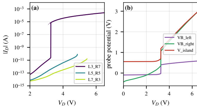
Fig. 7. Floating n^+ island (폭 30 nm). (a) 도핑 배치별 |I_D| . (b) L3 R7의 probe 전위: 래치 전에는 두 body가 다른 전위이지만 3.26 V에서 함께 점프한다. 데이터: 0928/ISL_W30_{L3_R7,L5_R5,L7_R3}.log.
