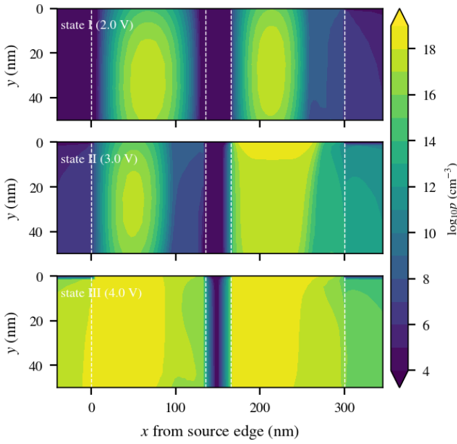
Fig. 15. 세 상태의 성공 밀도 \log_{10} p (기준 소자 up sweep; 점선: source 끝 0 nm, island 135–165 nm, drain 끝 300 nm). 상태 I: 두 body 모두 꺼짐. 상태 II: 오른쪽 body만 성공으로 채워짐. 상태 III: 두 body 모두 채워지고 island만 비어 있다. 데이터: 1007_ddsplit/DDS_BASE_SNAP_T_tr_N (.str, 스냅샷 번호: 1007_ddsplit/mech2_DD_SPLIT_BASE_SNAP.dat). 코드: paper/make_figs_ext.py, 1007_ddsplit/mech2_ddsplit.py.
