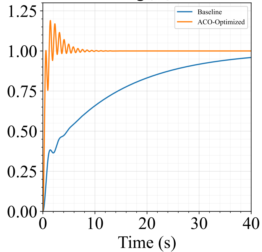
G_3(s)
