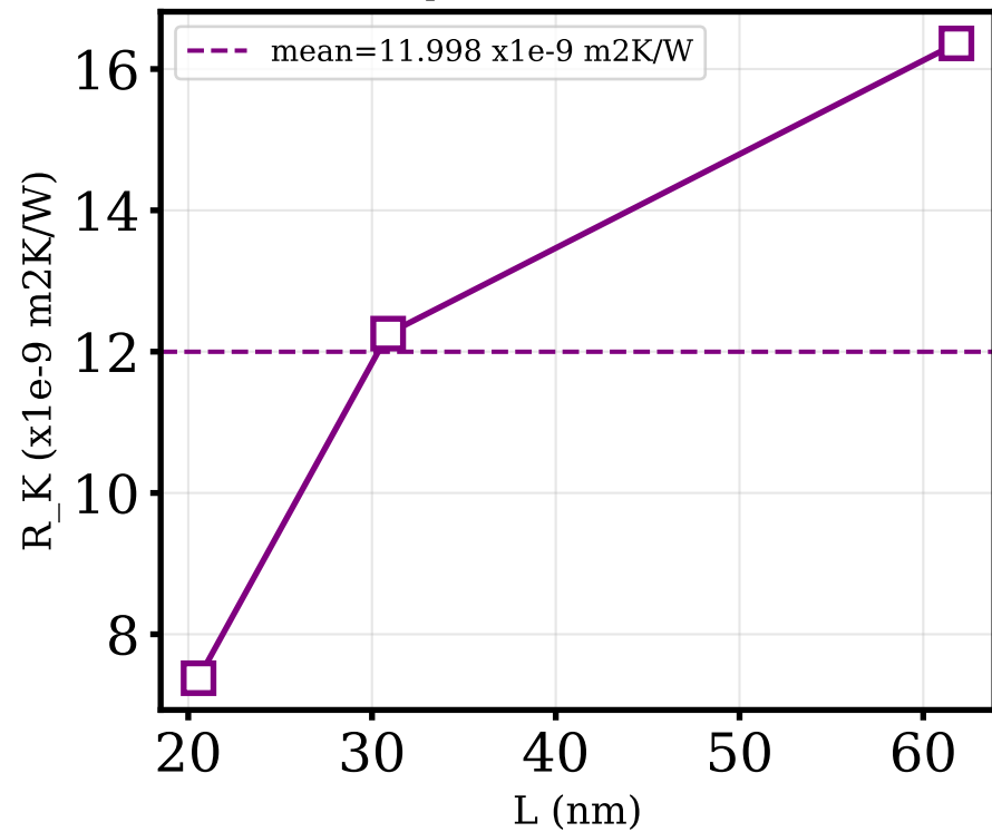
Kapitza Resistance vs L
