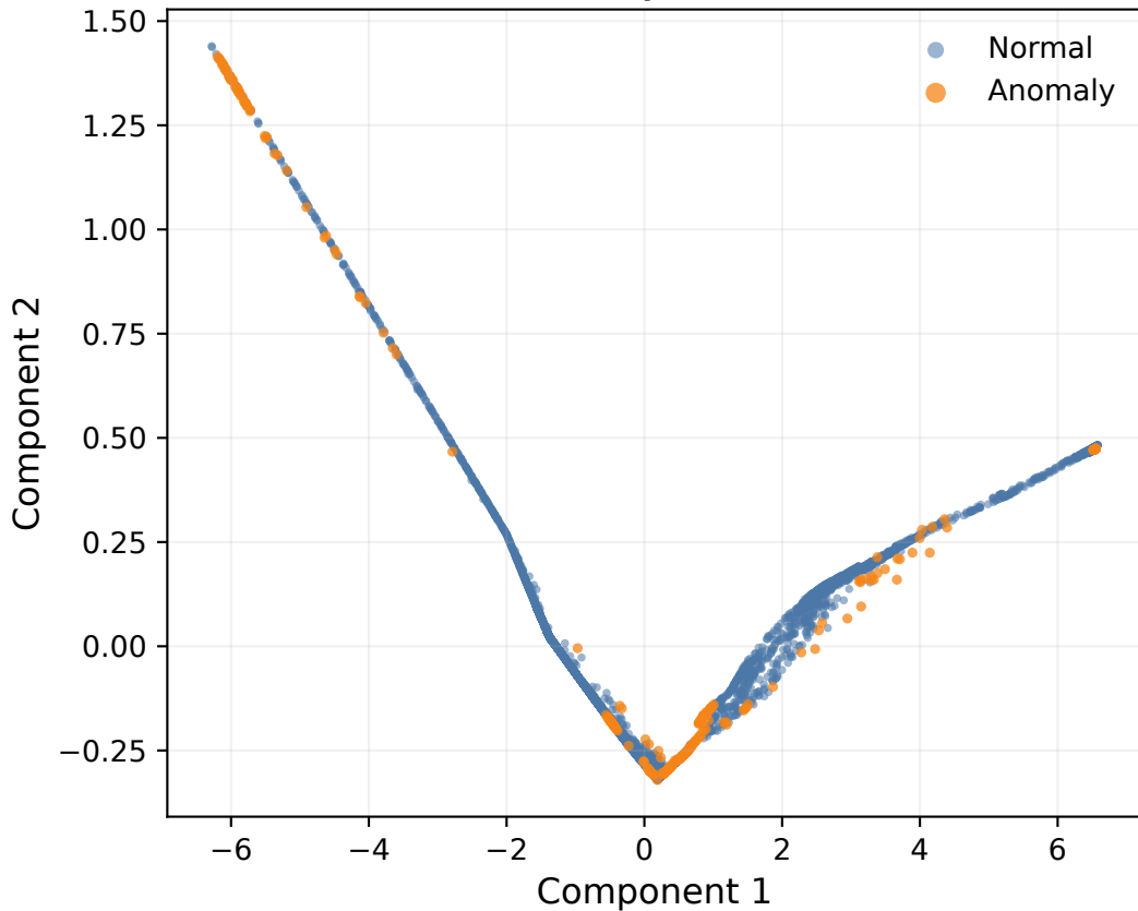
Latent PCA: Hybrid Quantum
