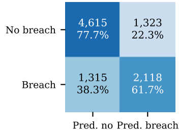
(d) Admissible, Random Forest
